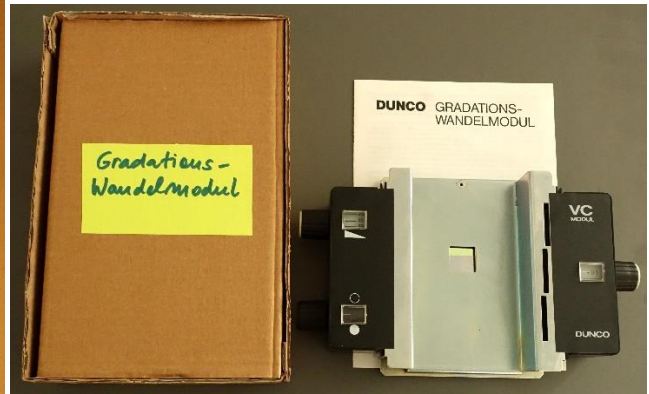
Gradationswandelmodul mit Originaverpackung
